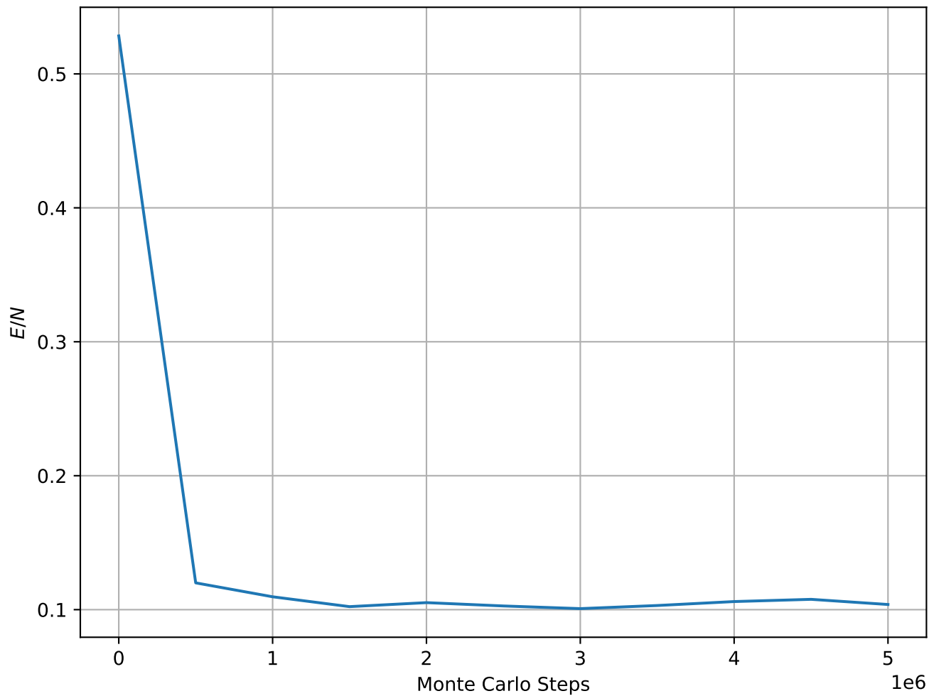
Energy per Spin at T = 8.00e - 02 , L = 32
