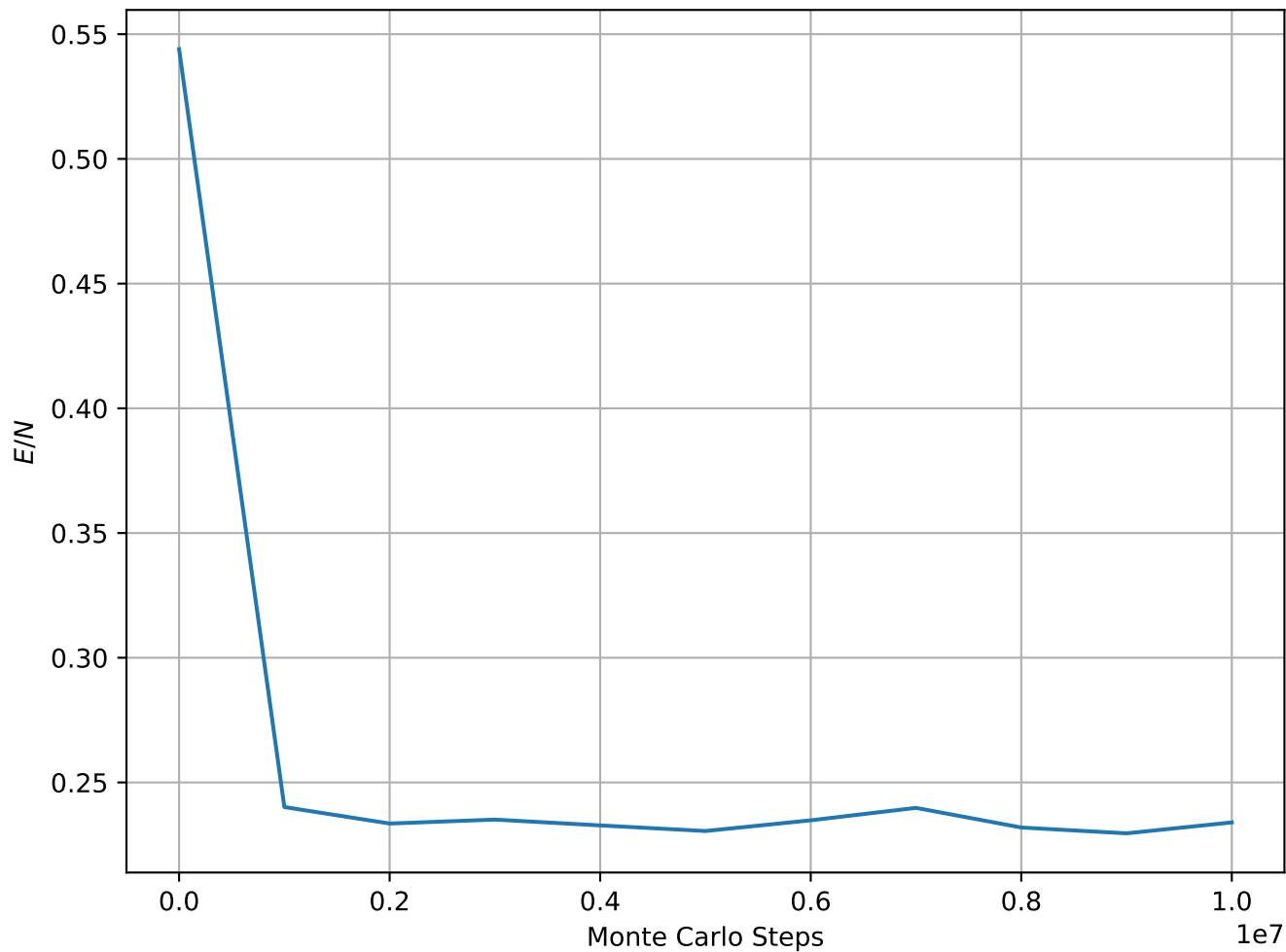
Energy per Spin at T = 1.60e - 01 , L = 64
