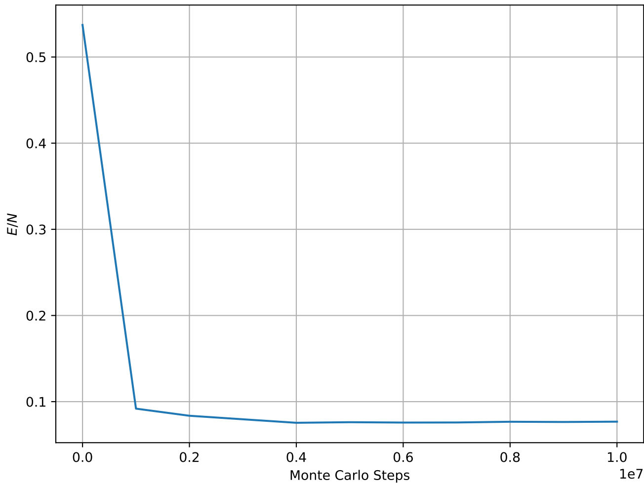
Energy per Spin at T = 6.00e - 02 , L = 64
