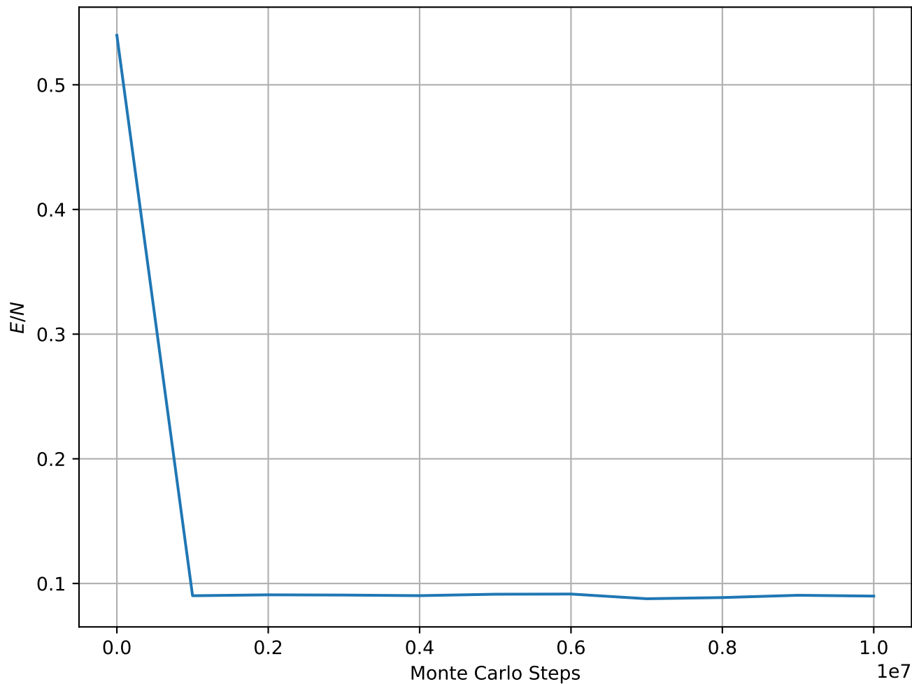
Energy per Spin at T = 7.00e - 02 , L = 64
