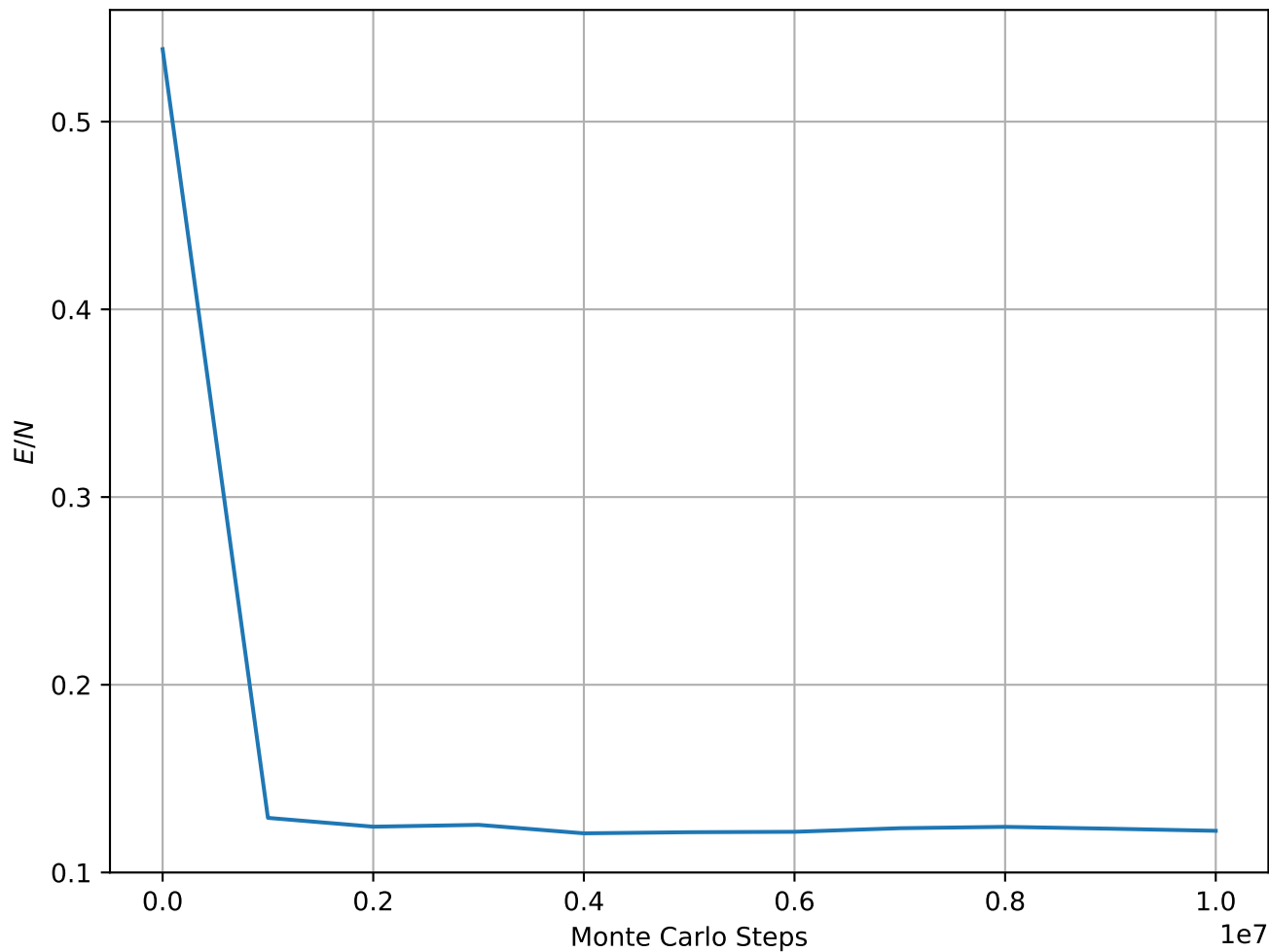
Energy per Spin at T = 9.00e - 02 , L = 64
