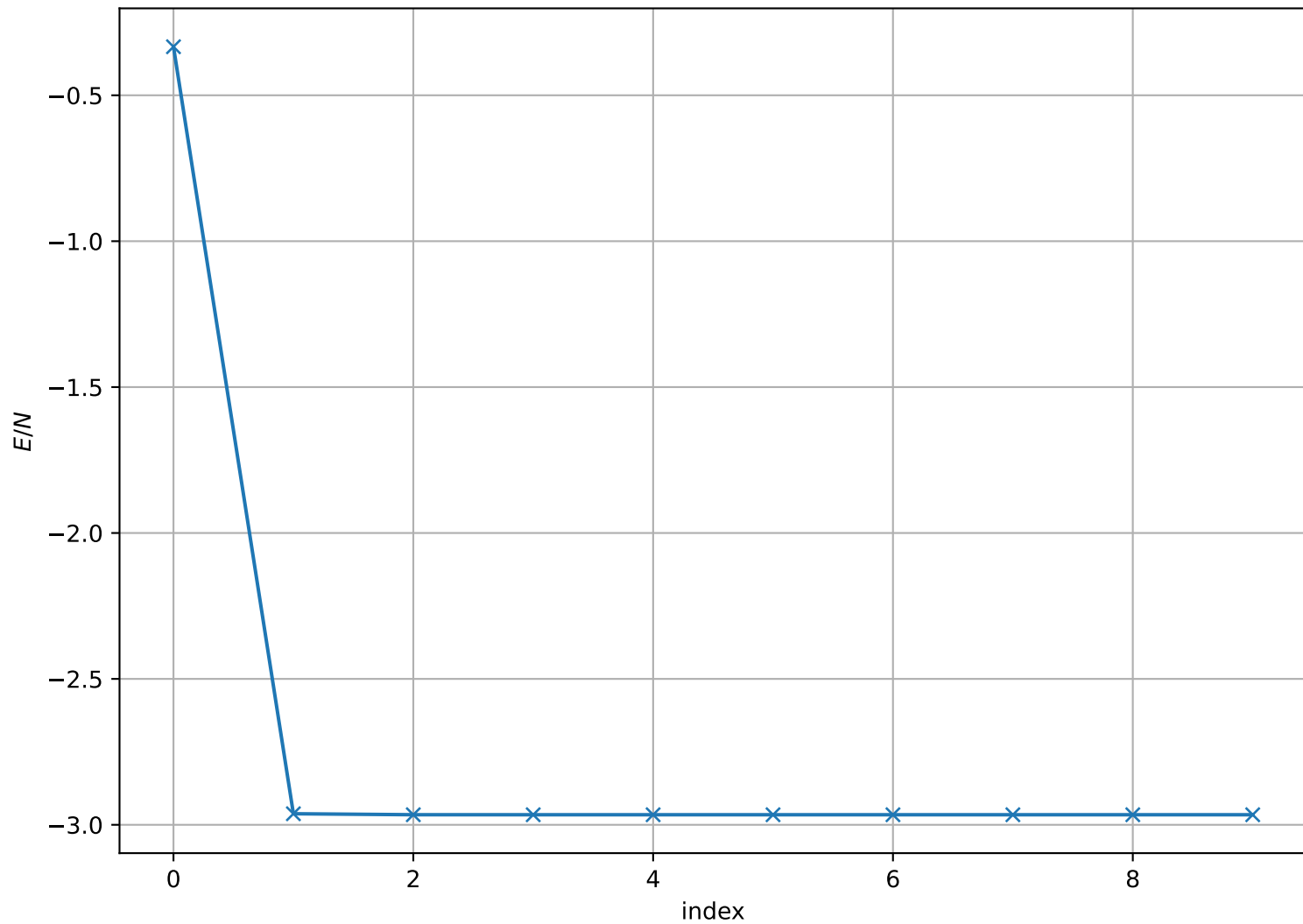
Energy per Site at T = 1.000\text{e} - 05 , L = 128
