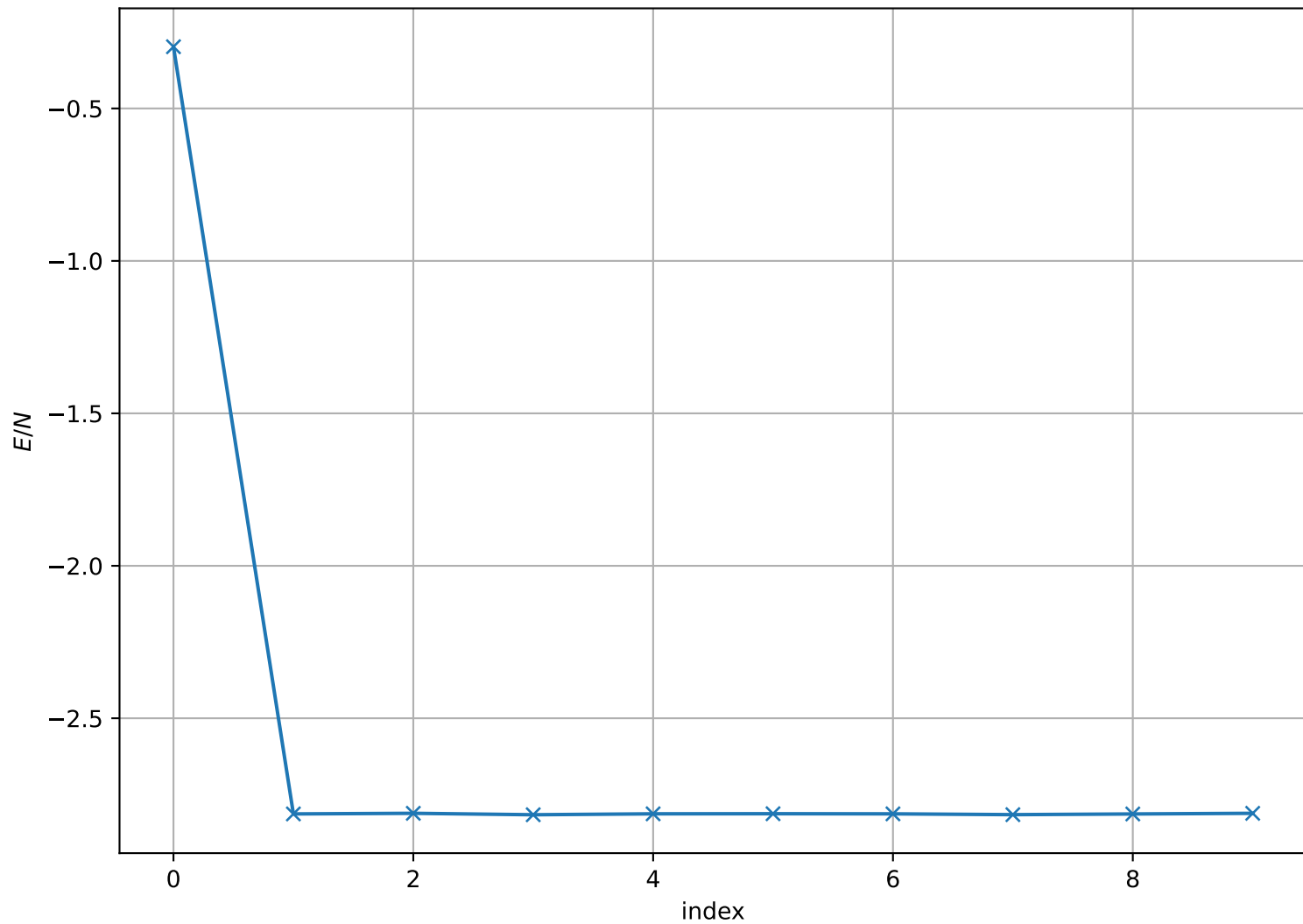
Energy per Site at T = 3.000e - 01 , L = 128
