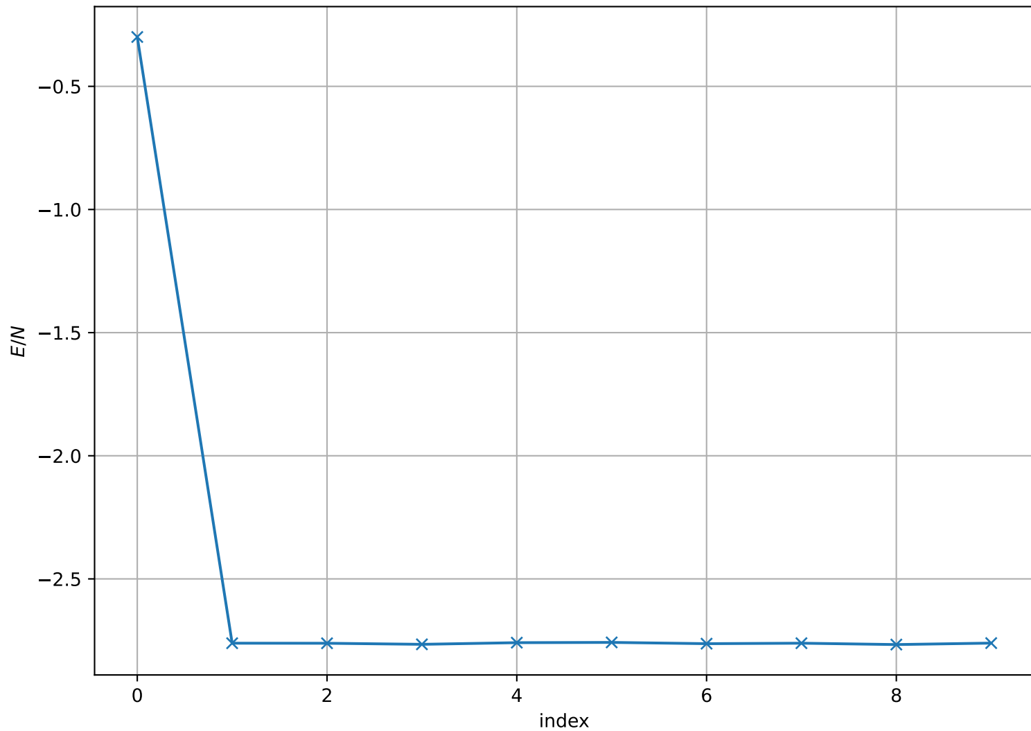
Energy per Site at T = 4.000e - 01 , L = 128
