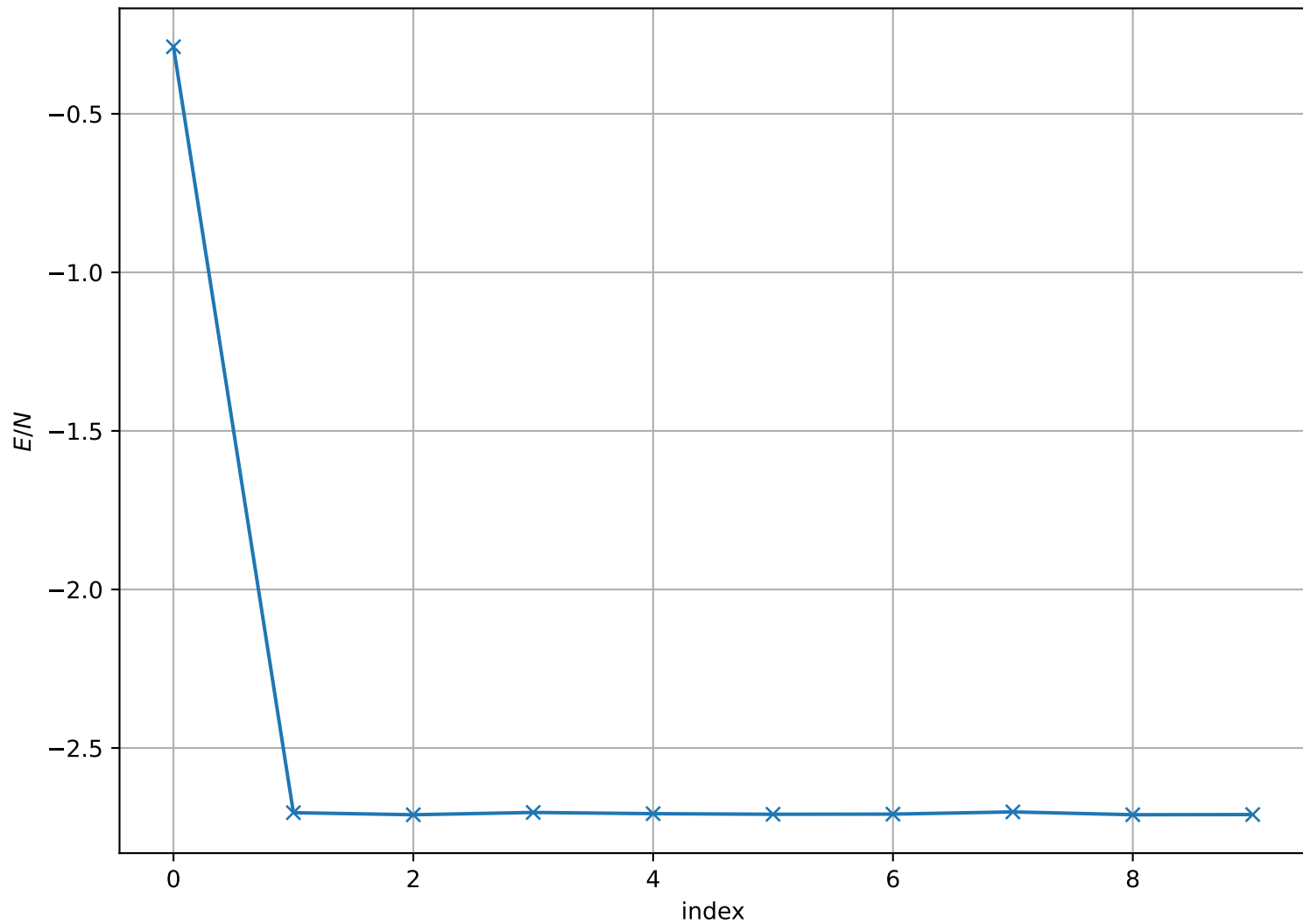
Energy per Site at T = 5.000e - 01 , L = 128
