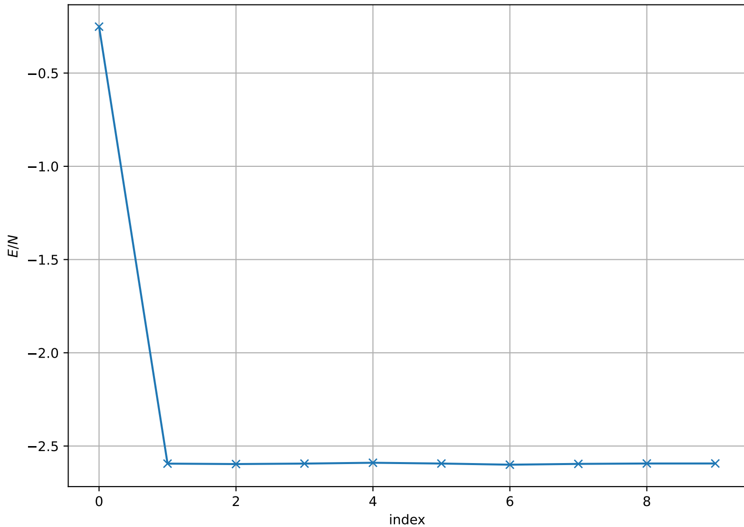
Energy per Site at T = 7.000e - 01 , L = 128
