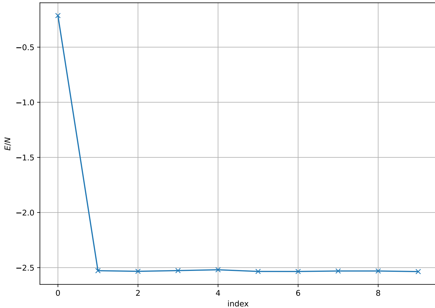
Energy per Site at T = 8.000e - 01 , L = 128
