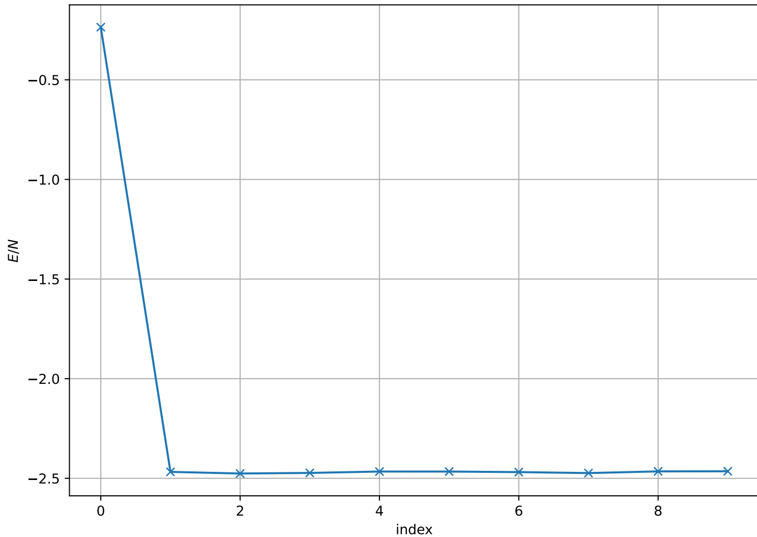
Energy per Site at T = 9.000e - 01 , L = 128
