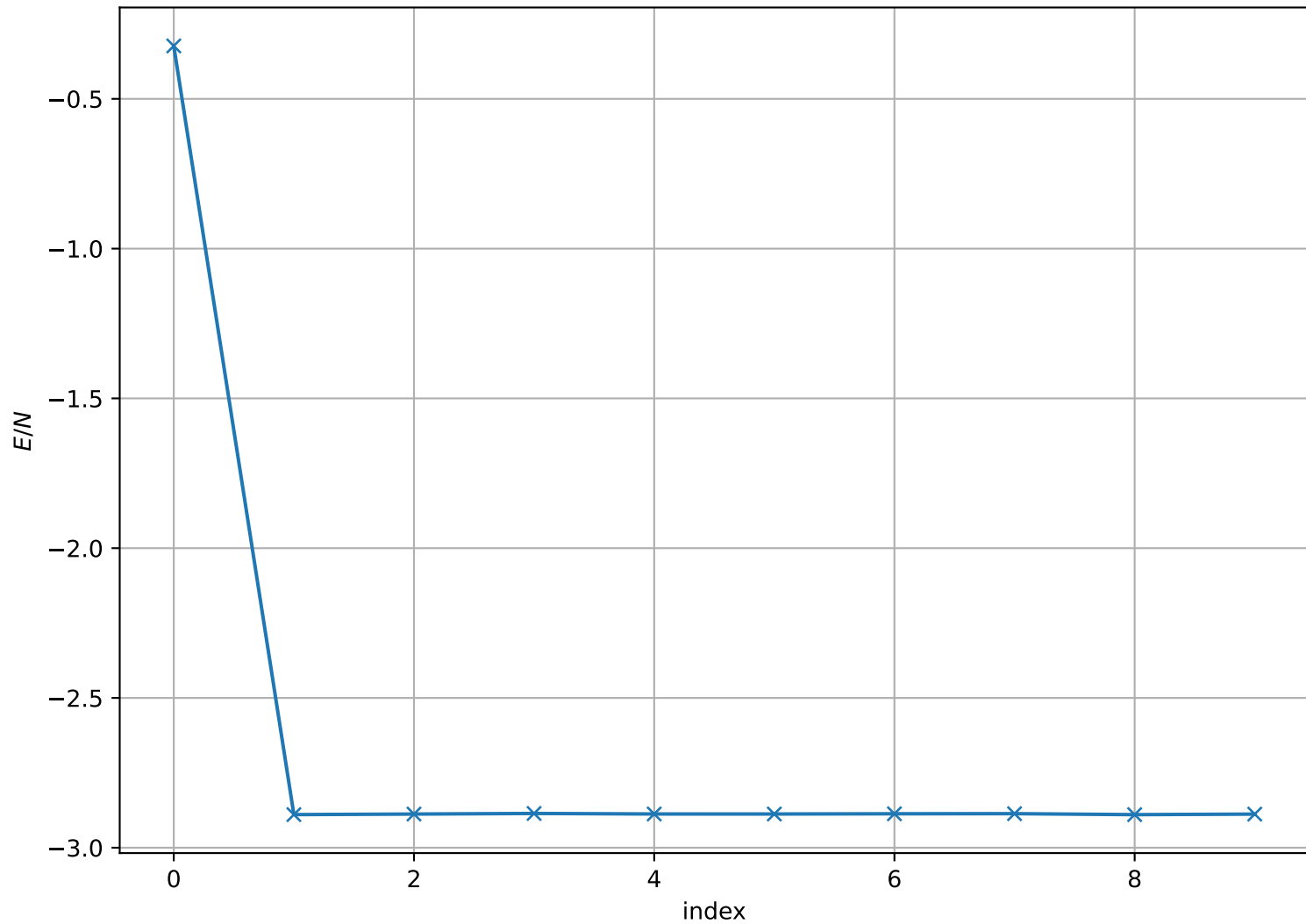
Energy per Site at T = 1.000e - 01 , L = 64
