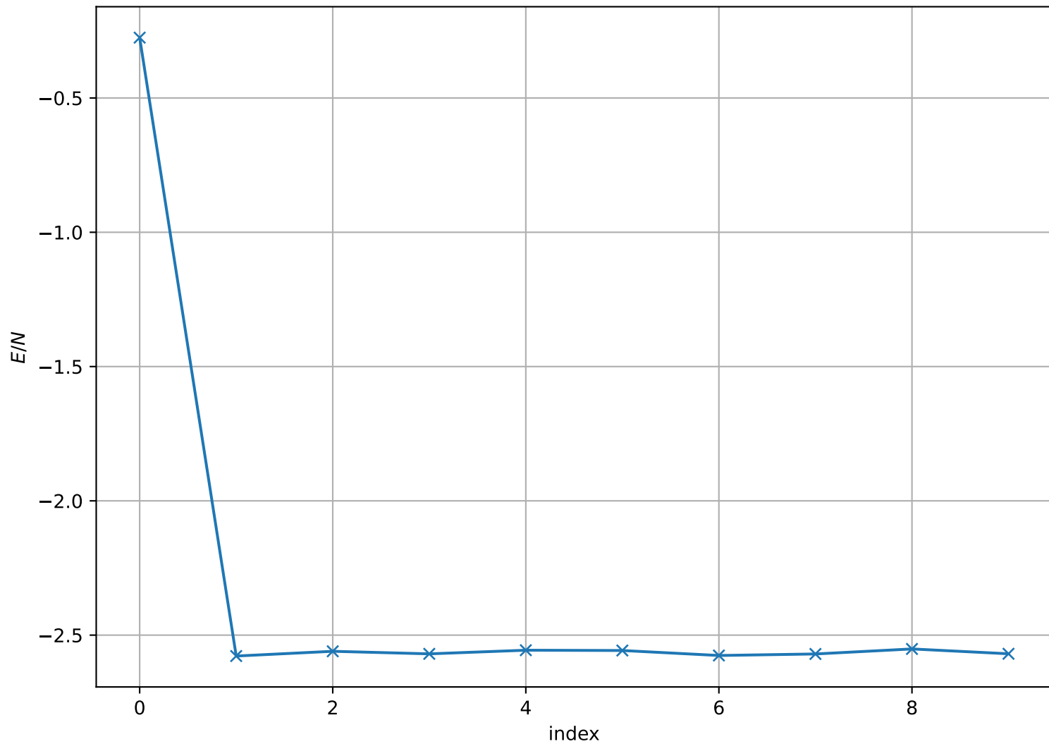
Energy per Site at T = 7.000e - 01 , L = 64
