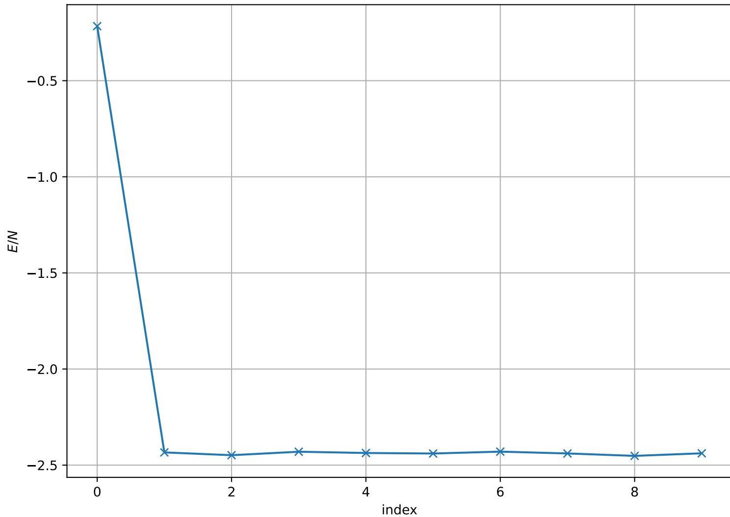
Energy per Site at T = 9.000e - 01 , L = 64
