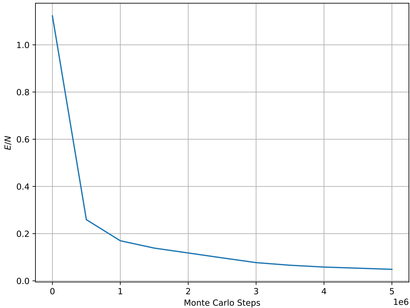
Energy per Spin at T = 1.00e - 02 , L = 128
