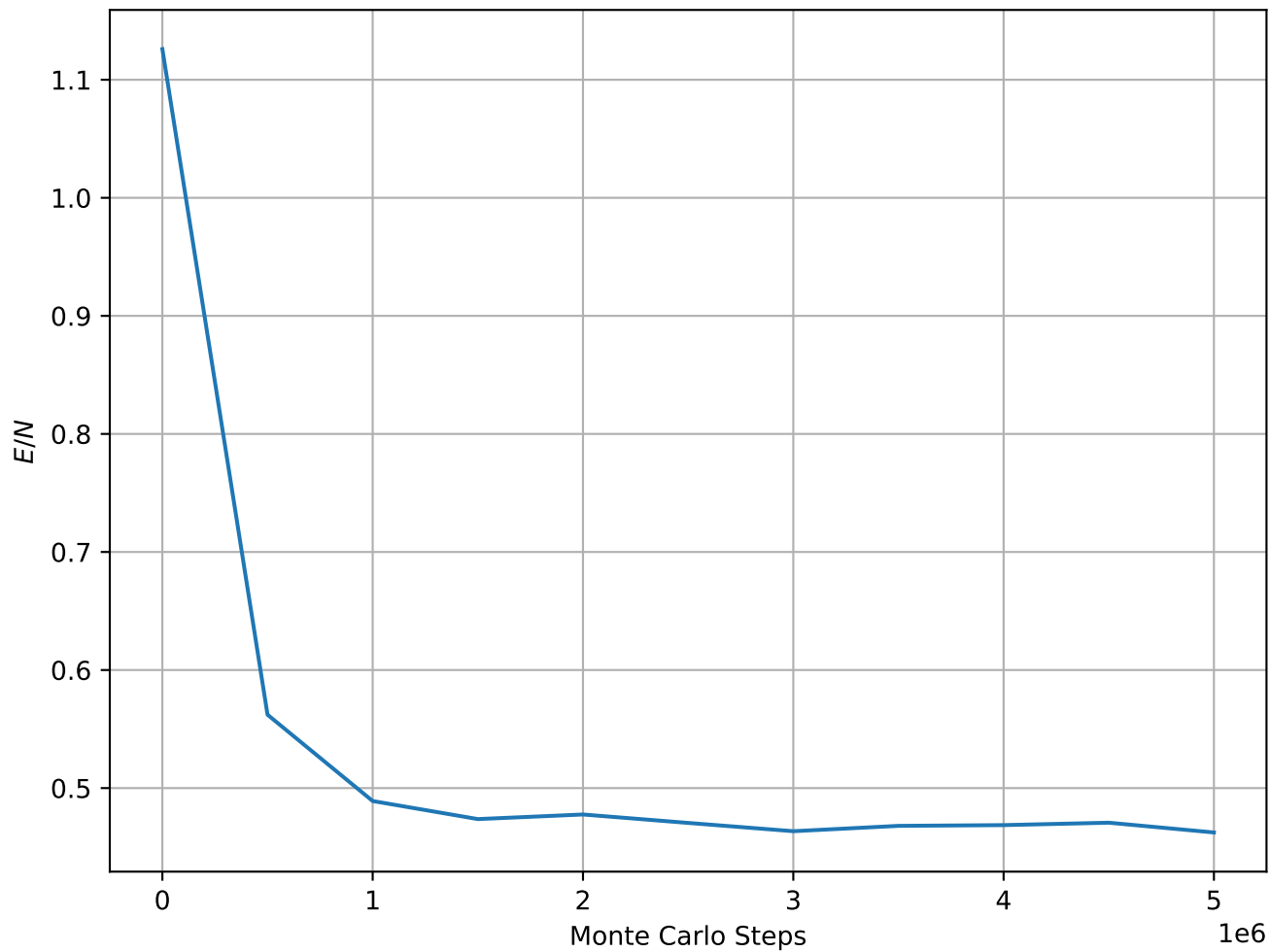
Energy per Spin at T = 1.50e - 01 , L = 128
