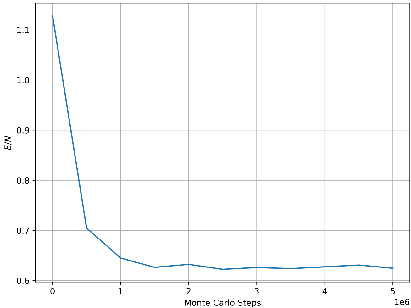
Energy per Spin at T = 1.90e - 01 , L = 128
