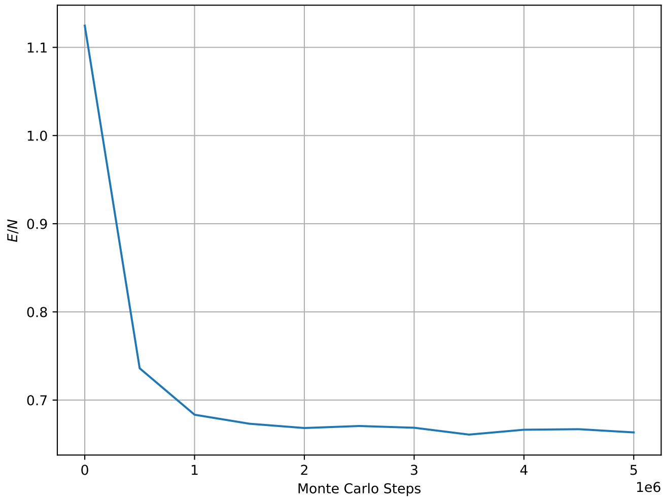
Energy per Spin at T = 1.96e - 01 , L = 128
