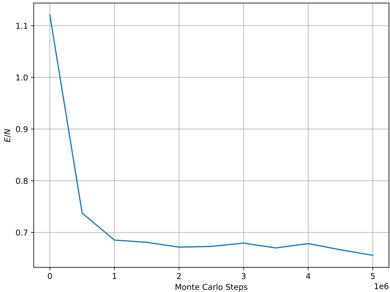
Energy per Spin at T = 1.97e - 01 , L = 128
