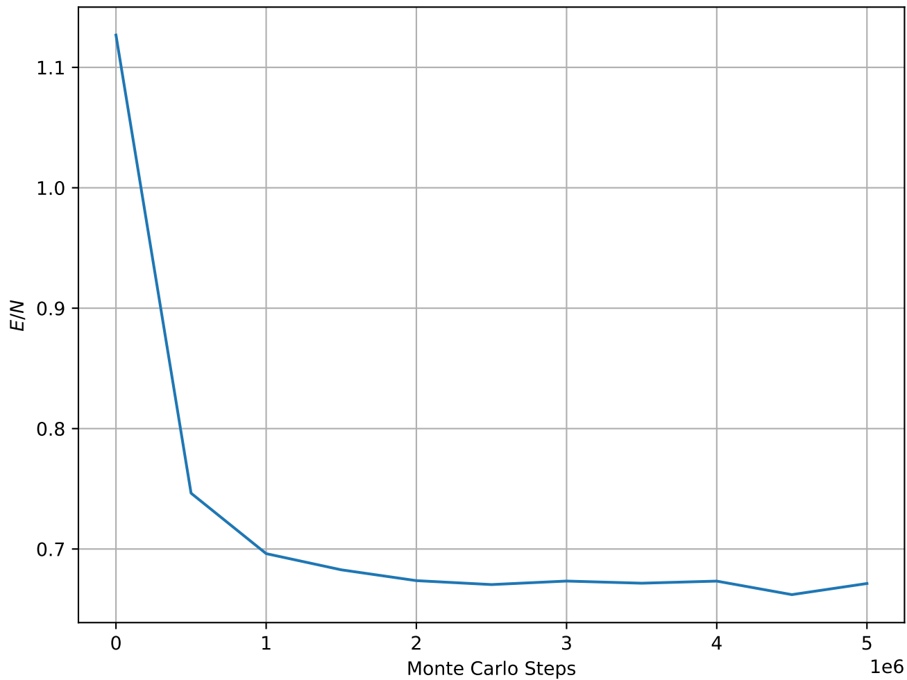
Energy per Spin at T = 1.98e - 01 , L = 128
