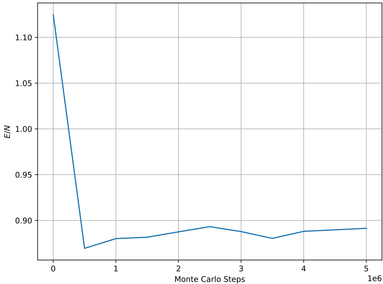
Energy per Spin at T = 2.50e - 01 , L = 128
