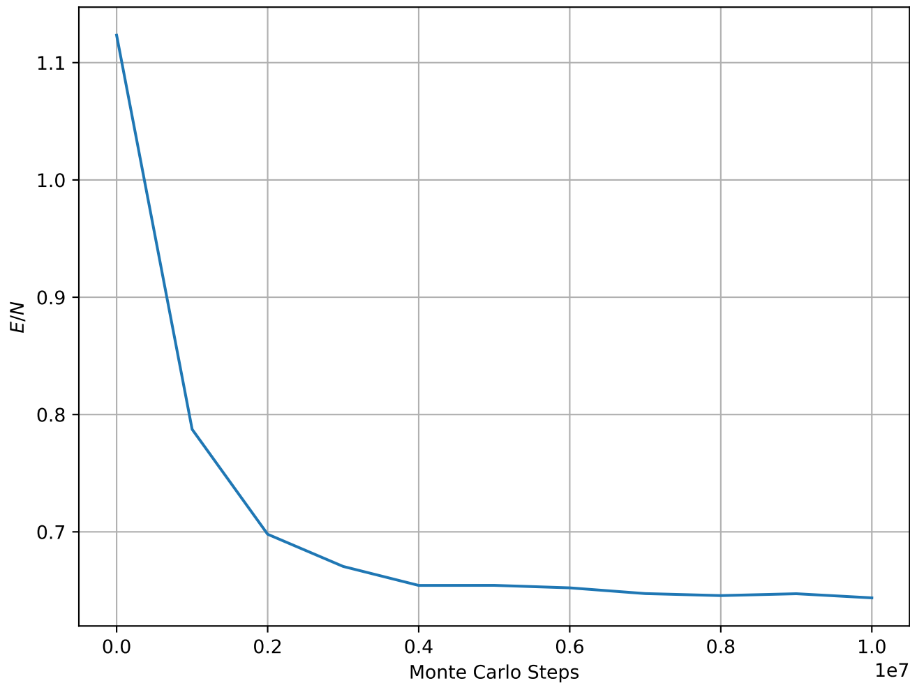
Energy per Spin at T = 1.90e - 01 , L = 256
