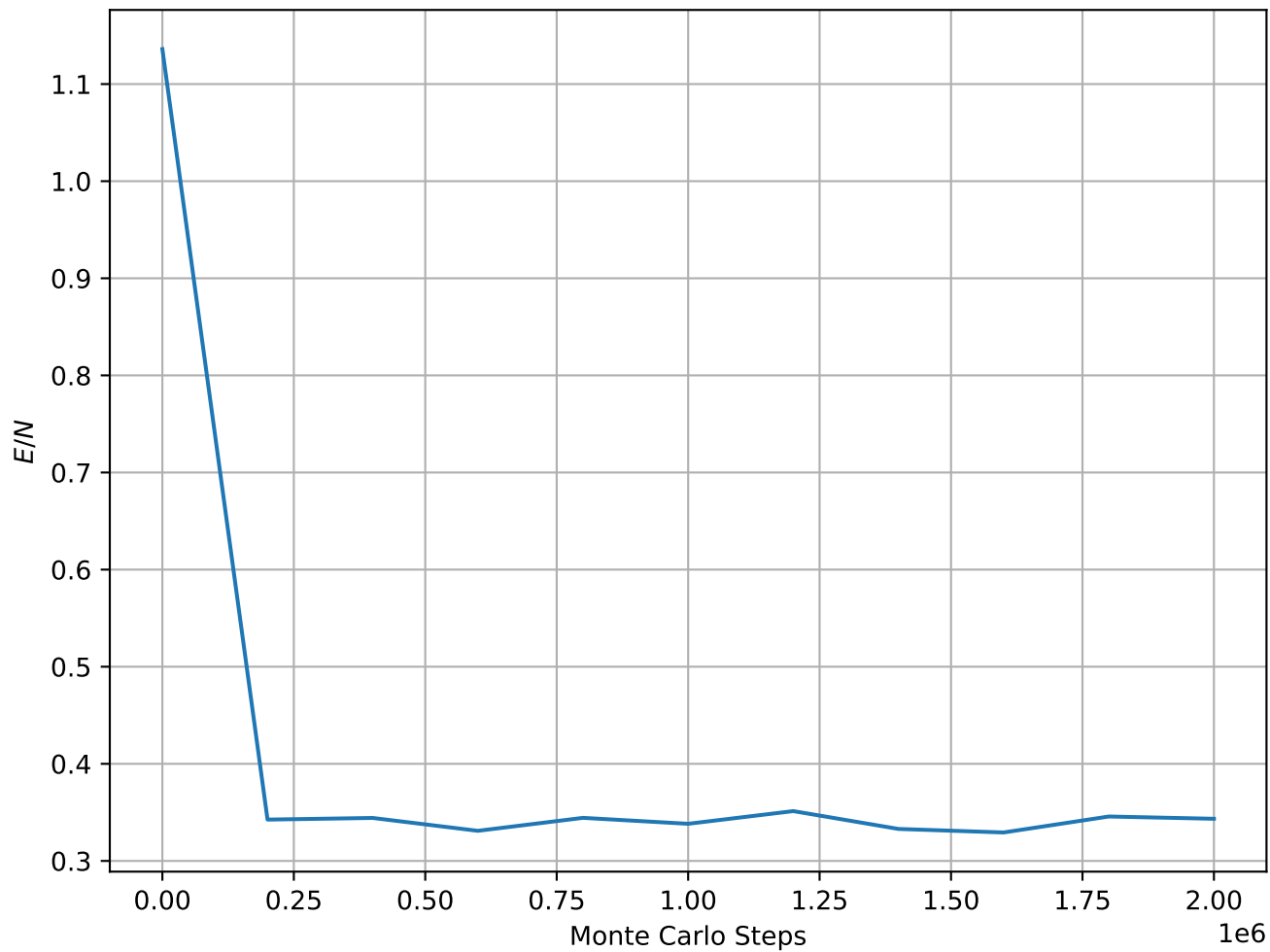
Energy per Spin at T = 1.20e - 01 , L = 32
