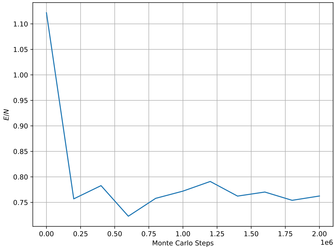
Energy per Spin at T = 2.20e - 01 , L = 32
