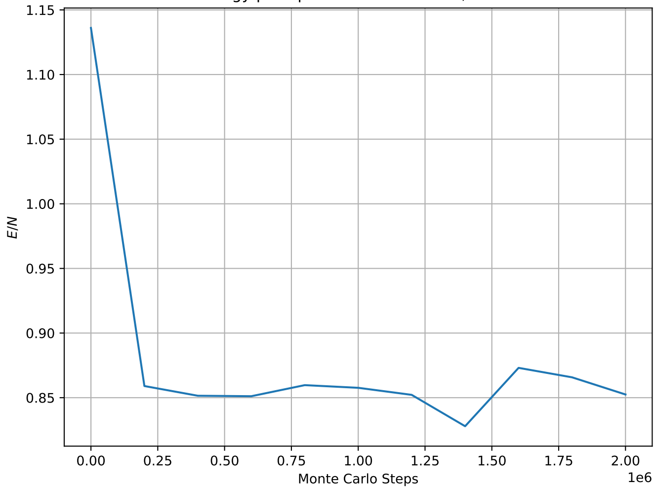
Energy per Spin at T = 2.50e - 01 , L = 32
