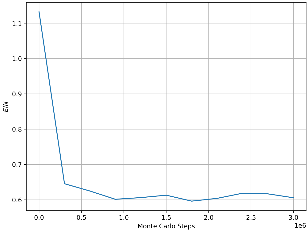
Energy per Spin at T = 1.90e - 01 , L = 64
