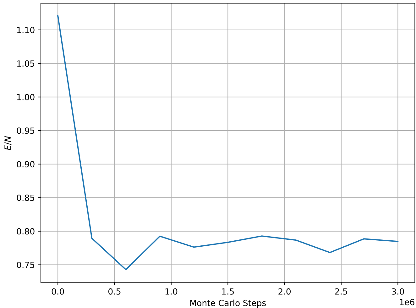
Energy per Spin at T = 2.20e - 01 , L = 64
