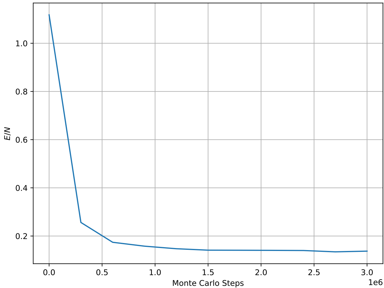
Energy per Spin at T = 5.00e - 02 , L = 64
