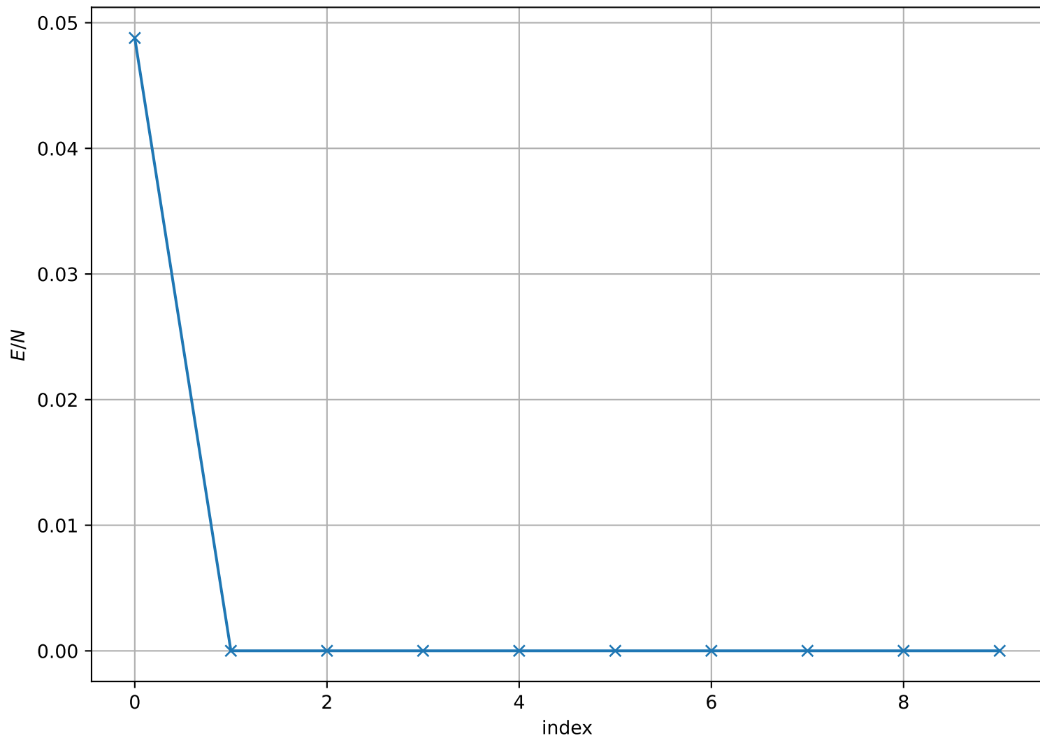
Energy per Site at T = 1.000e - 05 , L = 32
