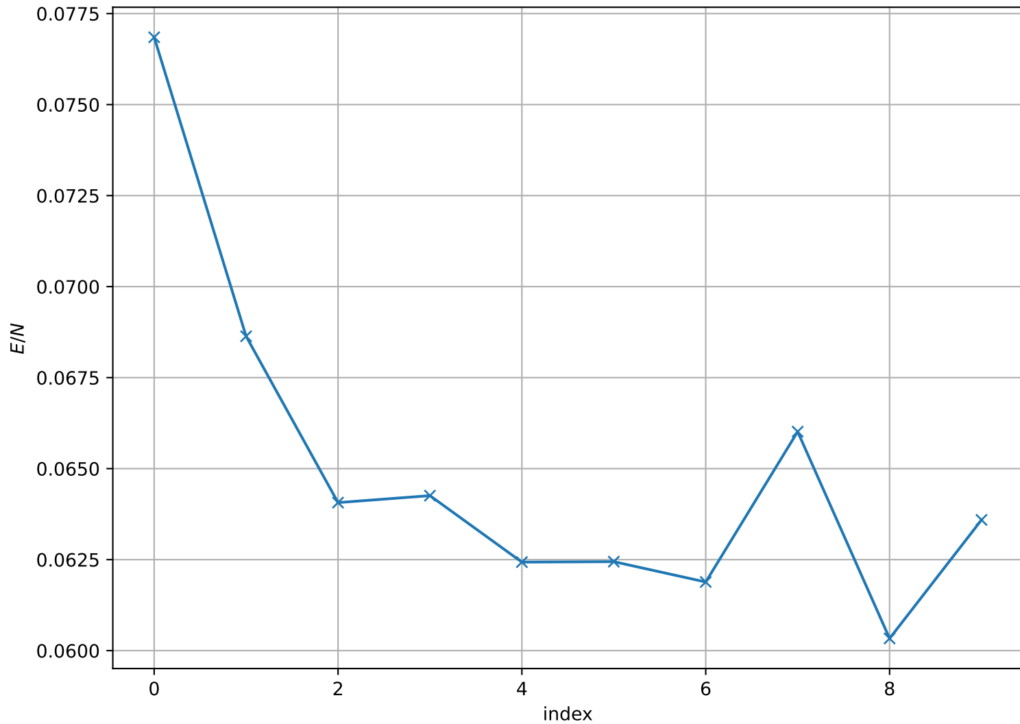
Energy per Site at T = 2.000e - 01 , L = 32
