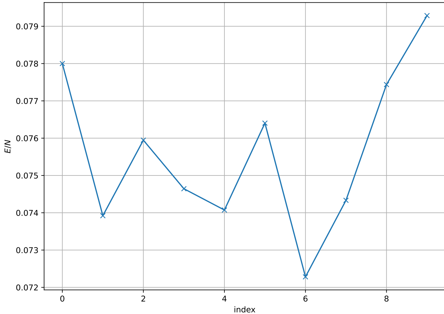
Energy per Site at T = 4.000e - 01 , L = 32
