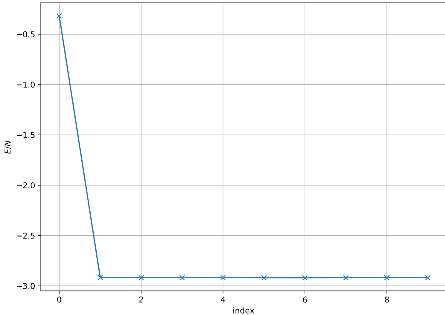
Energy per Site at T = 1.000e - 01 , L = 128
