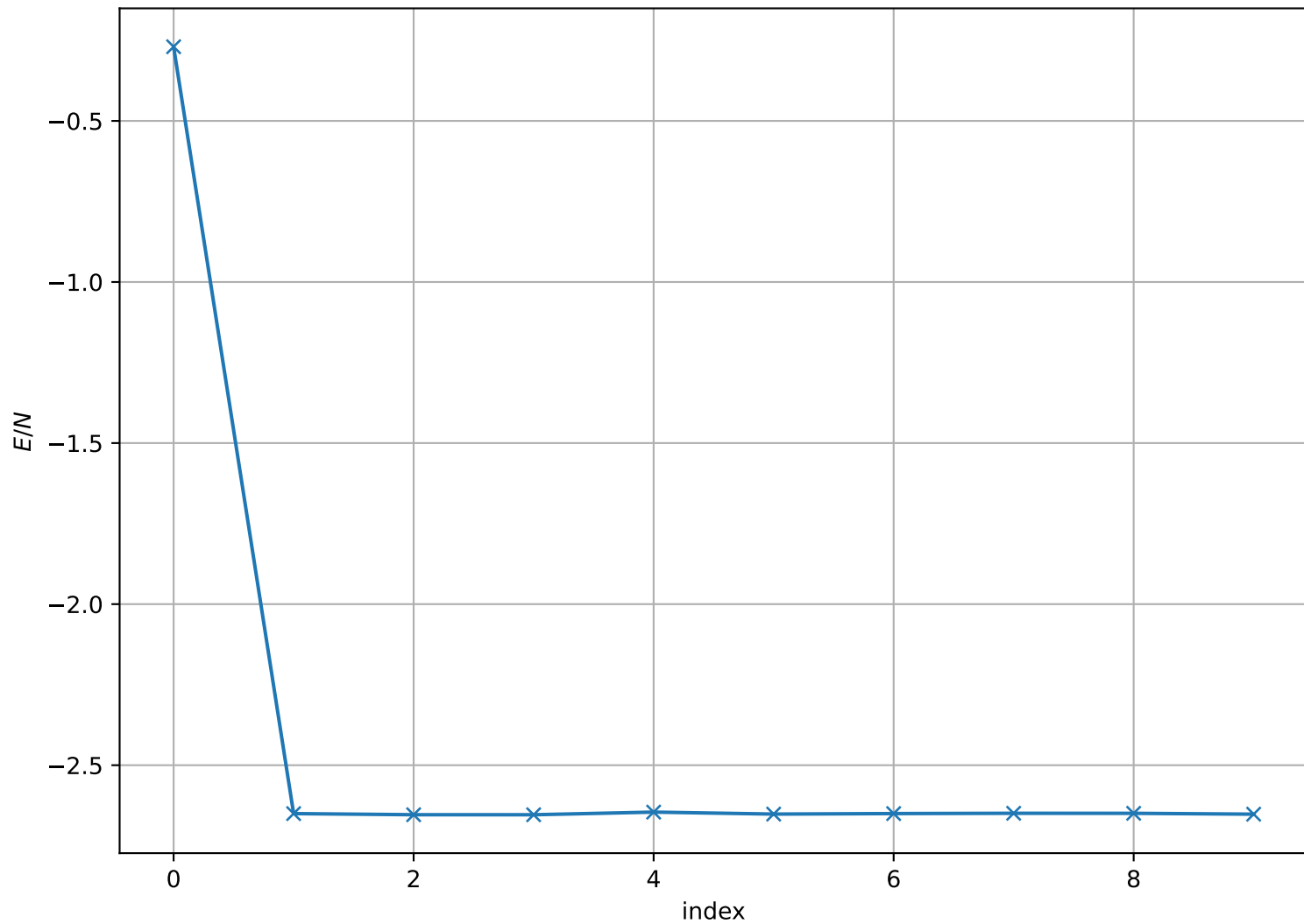
Energy per Site at T = 6.000e - 01 , L = 128
