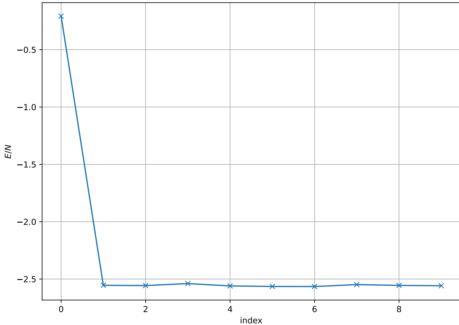
Energy per Site at T = 6.000e - 01 , L = 32
