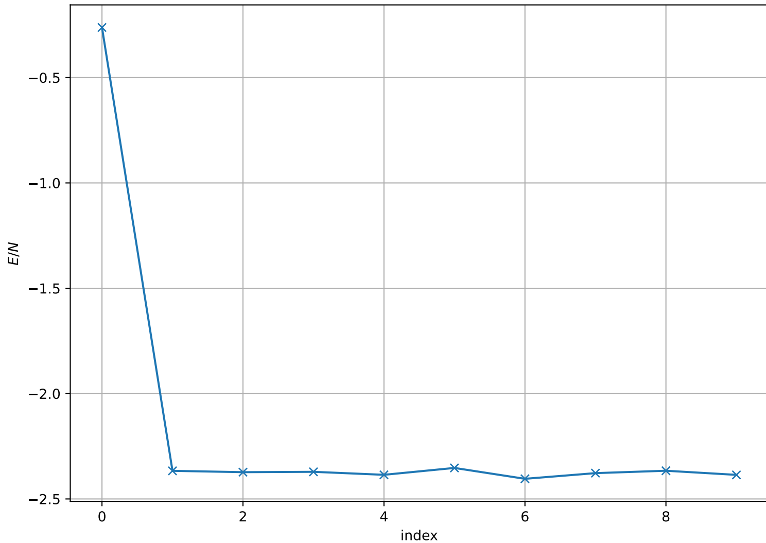
Energy per Site at T = 9.000e - 01 , L = 32
