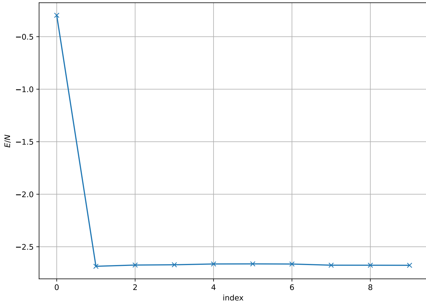
Energy per Site at T = 5.000e - 01 , L = 64
