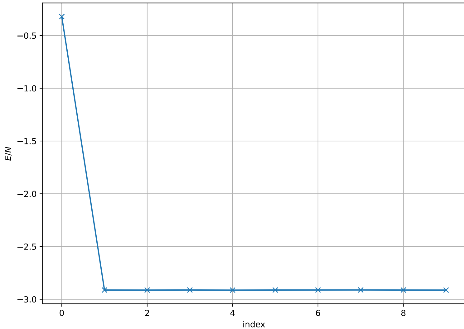
Energy per Site at T = 5.000e - 02 , L = 64
