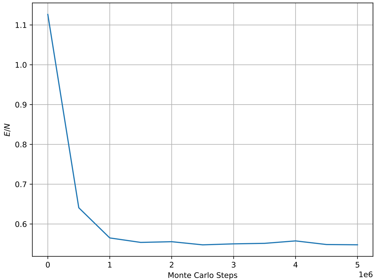
Energy per Spin at T = 1.70e - 01 , L = 128
