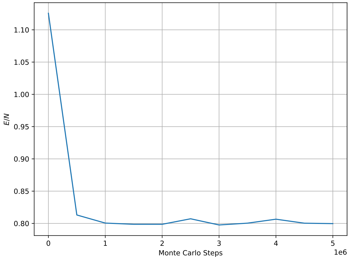
Energy per Spin at T = 2.20e - 01 , L = 128
