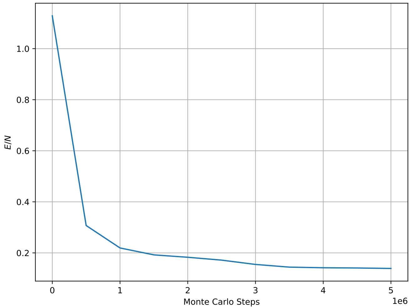
Energy per Spin at T = 5.00e - 02 , L = 128
