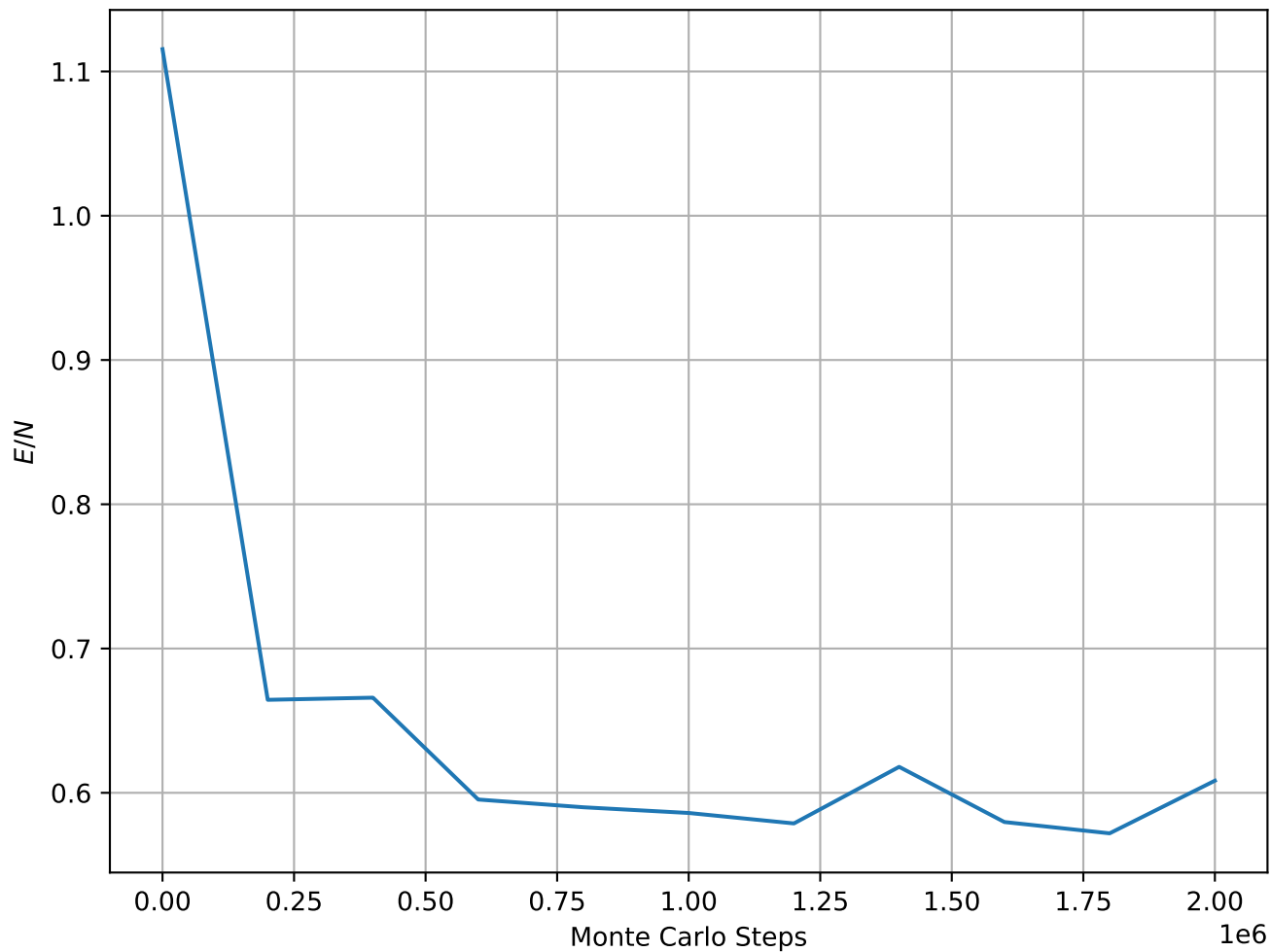
Energy per Spin at T = 1.90e - 01 , L = 32
