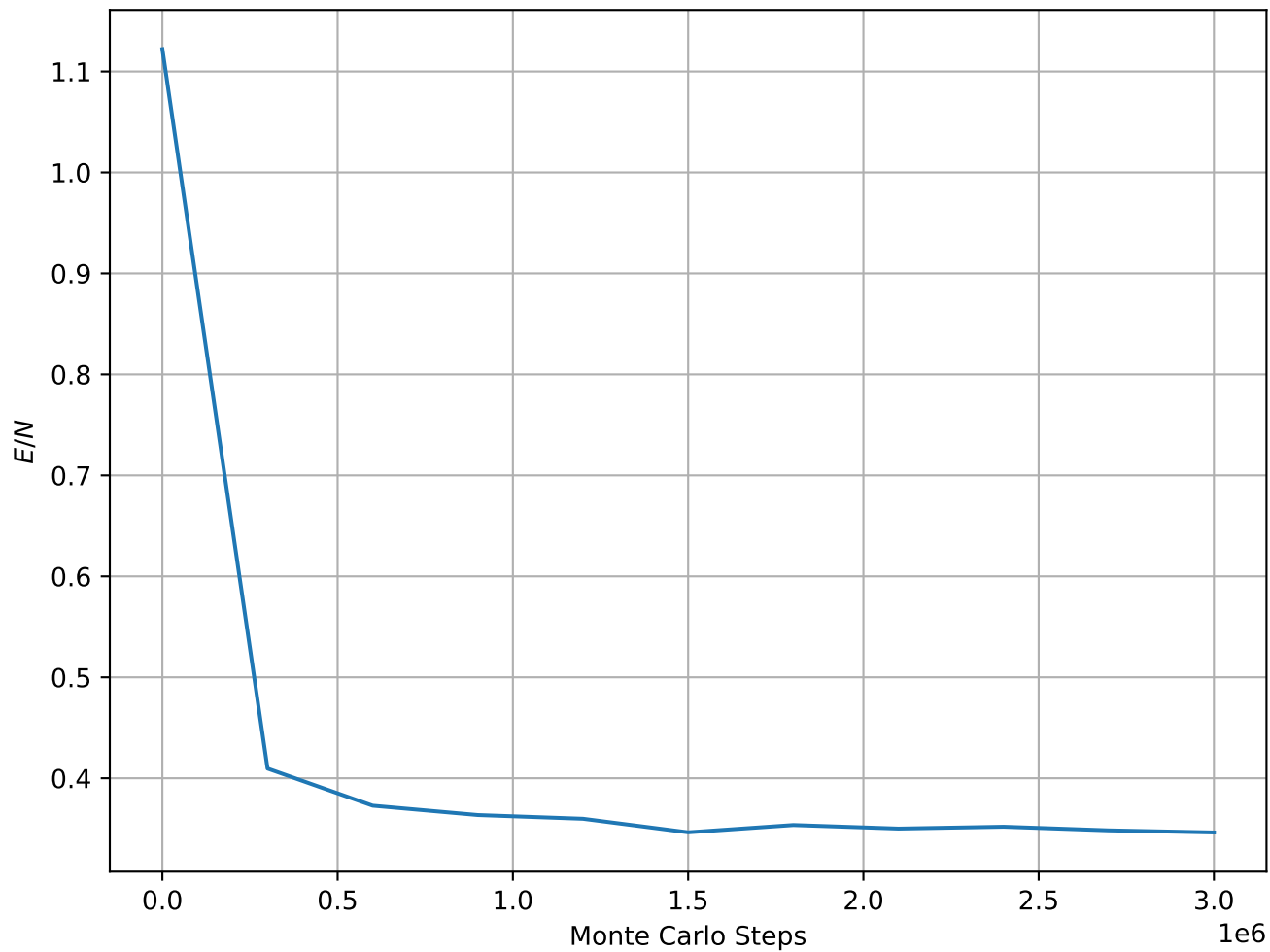
Energy per Spin at T = 1.20e - 01 , L = 64
