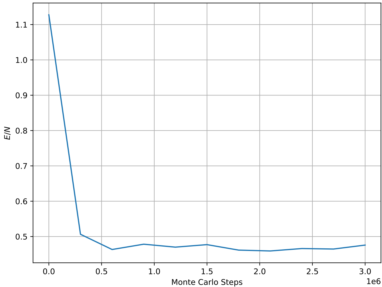
Energy per Spin at T = 1.50e - 01 , L = 64
