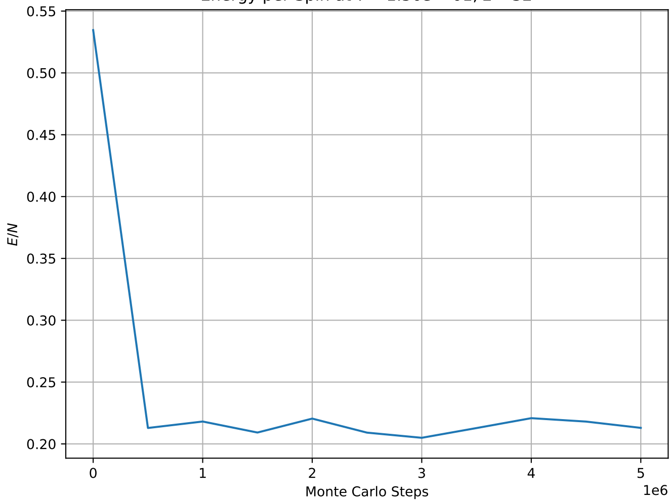
Energy per Spin at T = 1.50e - 01 , L = 32
