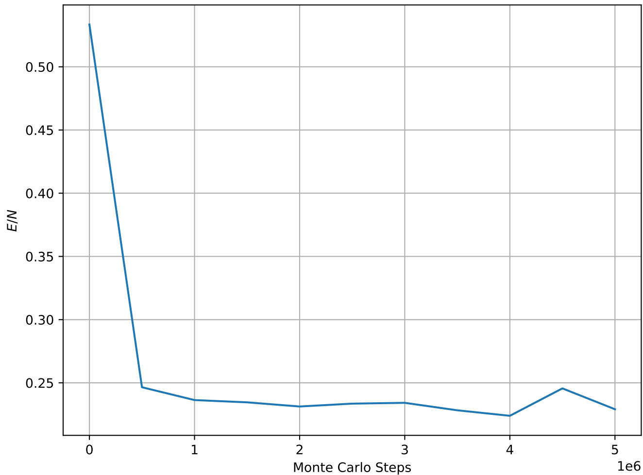
Energy per Spin at T = 1.60e - 01 , L = 32
