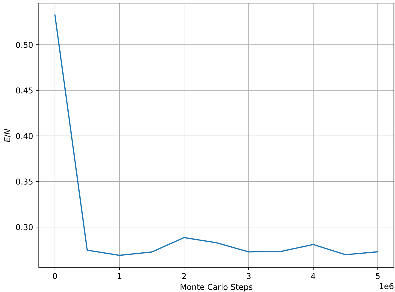
Energy per Spin at T = 1.80e - 01 , L = 32
