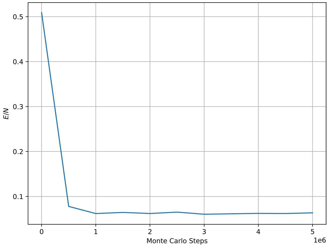
Energy per Spin at T = 5.00e - 02 , L = 32
