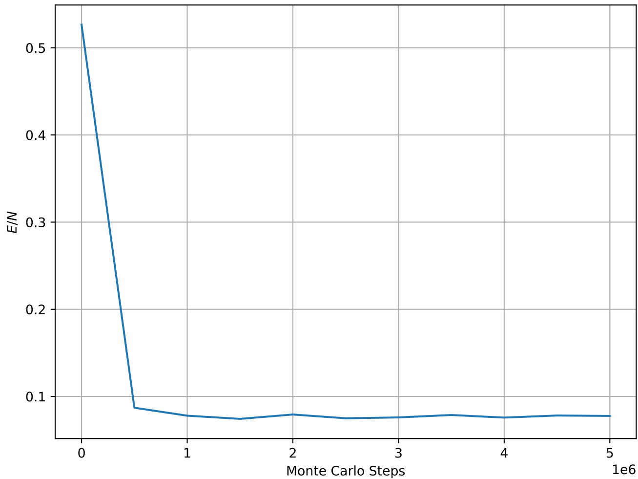
Energy per Spin at T = 6.00e - 02 , L = 32
