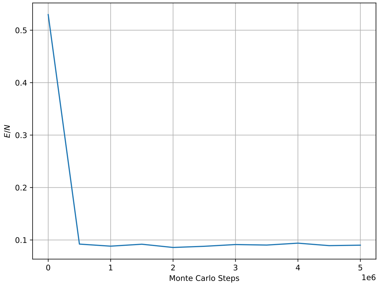
Energy per Spin at T = 7.00e - 02 , L = 32
